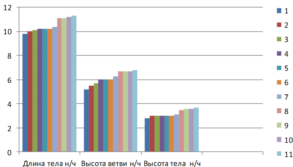
Рис. 1. Возрастная изменчивость тела и ветви нижней челюсти: 1 – семилетние; 2 – восьмилетние; 3 – девятилетние; 4 – десятилетние; 5 – одиннадцатилетние; 6 – двенадцатилетние; 7 – тринадцатилетние; 8 – четырнадцатилетние; 9 – пятнадцатилетние; 10 – шестнадцатилетние; 11 – семнадцатилетние
